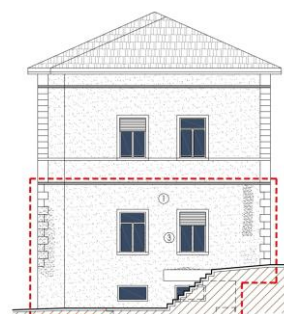
STATO DI PROGETTO PROSPETTO NORD-EST Scala 1:100
