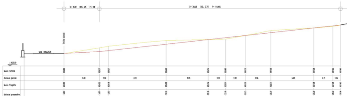
PROFILO LONGITUDINALE Scala 1:100
